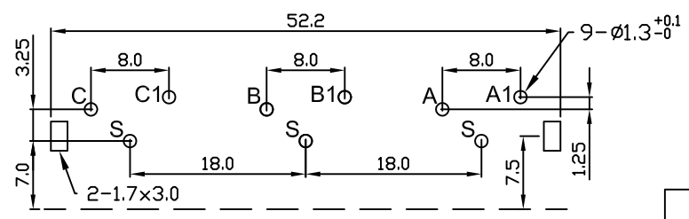
P.C.B LAYOUT(±0.1) (BOTTOM VIEW)
